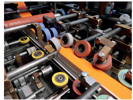
Die Flexibilität der Folie lässt es zu, auch Profile mit einem Kantenradius von lediglich einem Millimeter zu beschichten.
